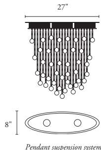
Pendant suspension system
